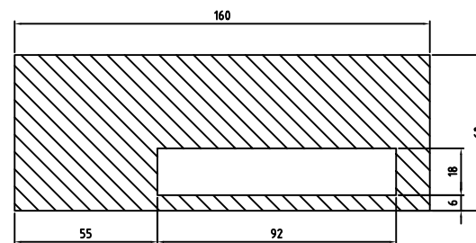
Страничен десен панел (изглед отпред)
